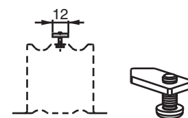
DH 220 - Holder into Heluz 220 lintel
